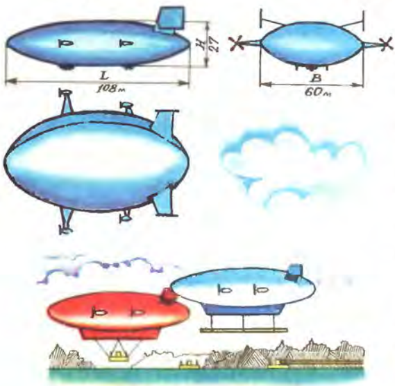
Компоновочная схема АКЛА, разработанного в Уральском общественном конструкторском бюро дирижаблестроения и пневмоконструций совместно с Уральским комплексным опытно-конструкторским отделом Всесоюзного института «Оргэнергострой».
