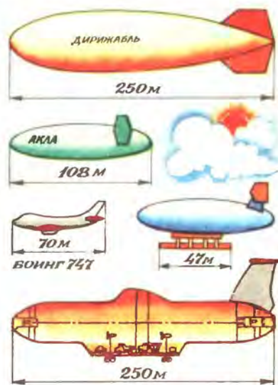
Компоновочная схема АКЛА, разработанного в Уральском общественном конструкторском бюро дирижаблестроения и пневмоконструций совместно с Уральским комплексным опытно-конструкторским отделом Всесоюзного института «Оргэнергострой».
