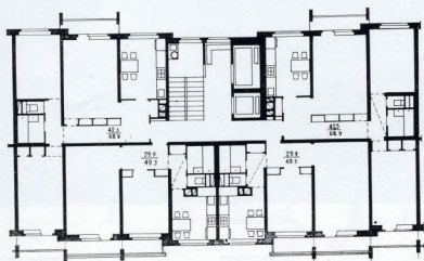
Шестнадцатизэтажный 256-квартирный панельный жилой дом П 3/16. Мастерская № 3. Руководитель А. Самсонов Макет и рядовая секция типового этажа, примеры блокировки секций
